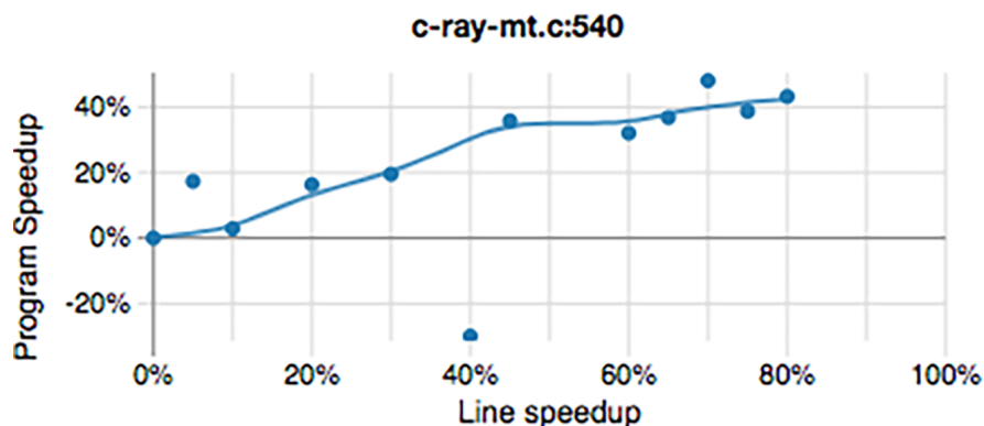
Figure 83: CozProfile 适用于 C-Ray 基准的 Coz 分析文件。
