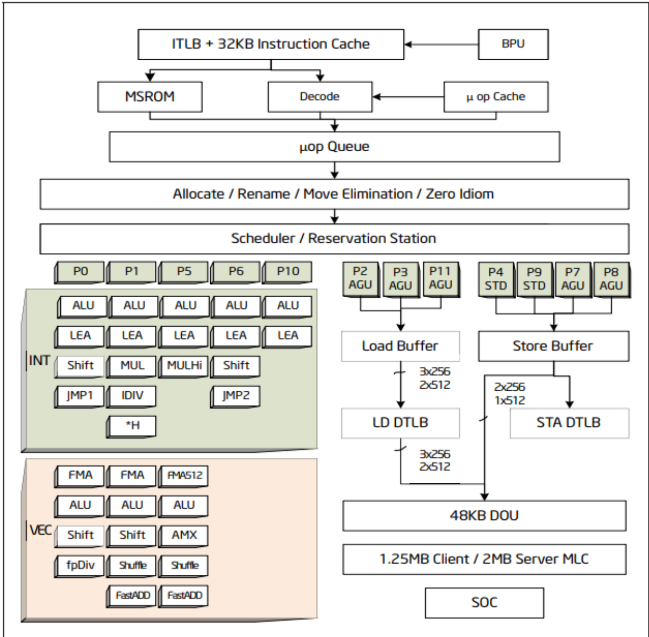
Figure 21: Intel GoldenCove 微架构 CPU 核心的模块图。© 图片来源 [Intel, 2023b]。
