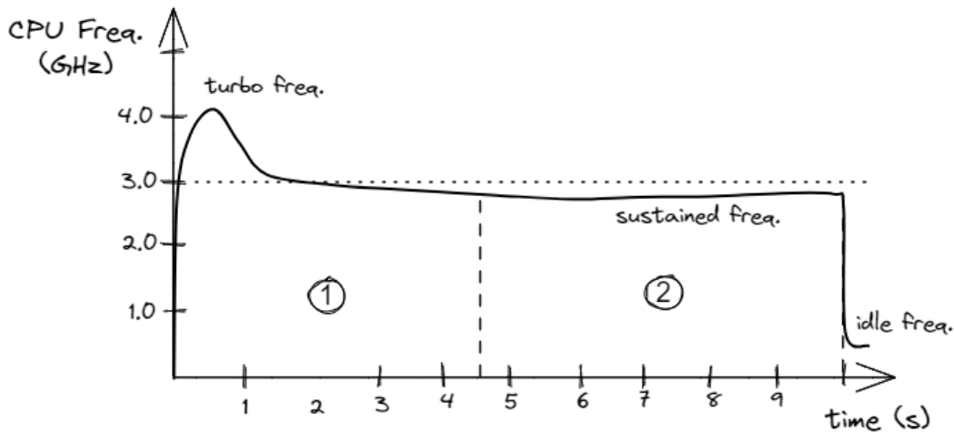
Figure 2: 频率缩放导致性能变化的差异：第一次运行比第二次运行快 1 秒。
