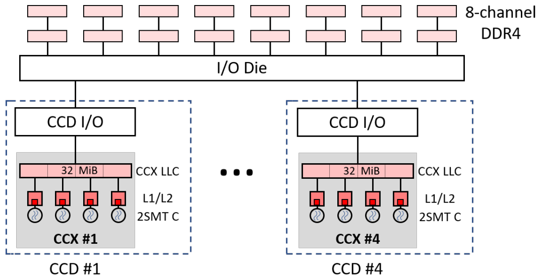
Figure 73: AMD Milan 7313P 处理器的集群式内存层次结构
