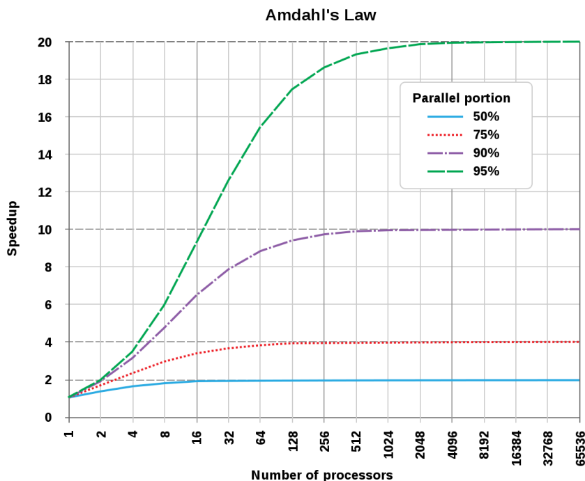
Figure 75: 根据安达尔定律，程序执行的理论加速度随处理器数量的变化。© Image by Daniels220 via Wikipedia.
