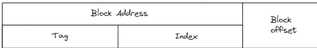
Figure 14: 用于缓存查找的地址组织。
