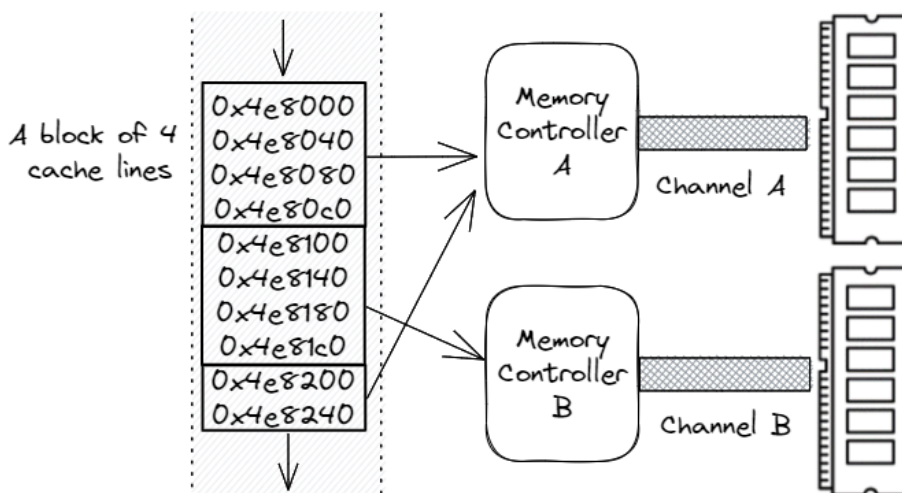
Figure 17: 顺序内存访问的 2 路交错。
