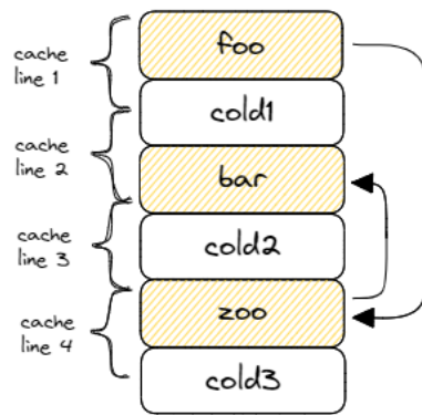
(a) 默认布局
