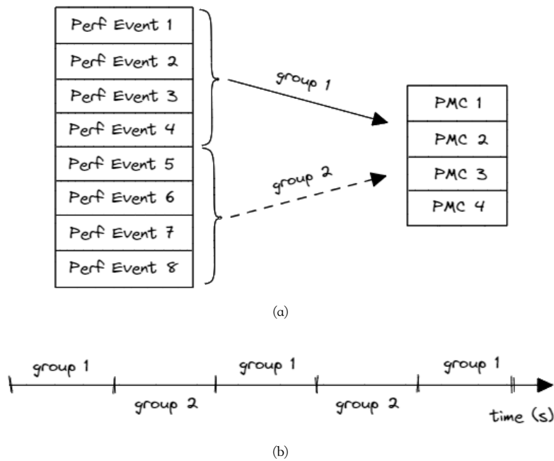
Figure 30: 8 个性能事件之间的多路复用示例，只有 4 个 PMC 可用。
