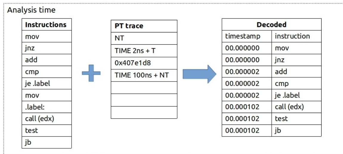
Figure 88: Intel 处理器跟踪时间数据包
