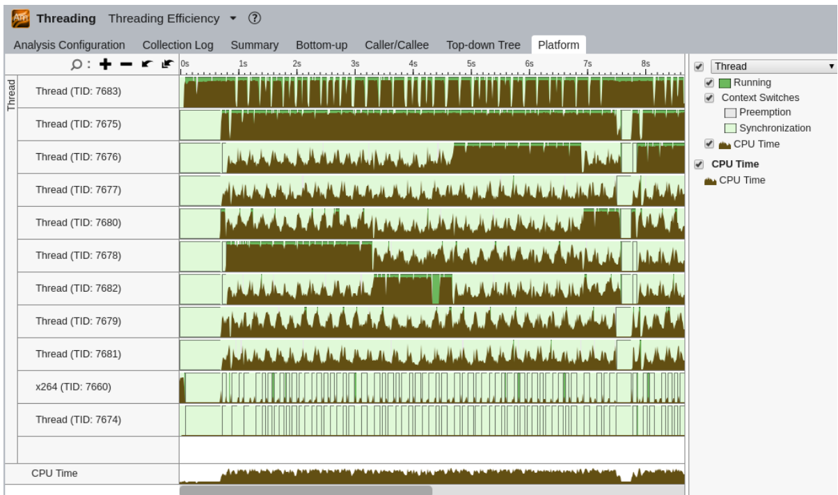
Figure 82: 显示了 Phoronix 测试套件中 x264 基准测试的 Intel VTune Profiler 平台视图。
