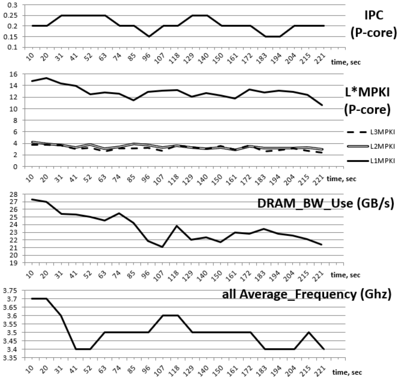
Figure 28: CloverLeaf 基准测试的一组指标图表
