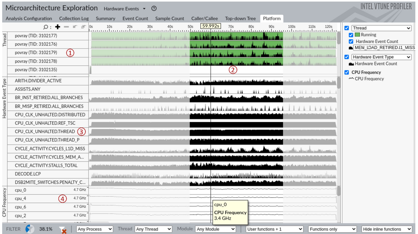
Figure 45: VTune 对 povray 内置基准测试的性能事件时间轴视图。
