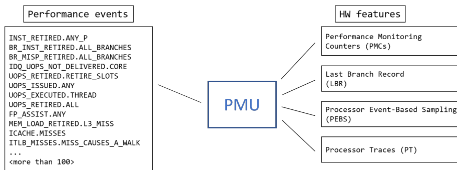
Figure 23: 现代 Intel CPU 的性能监控单元
