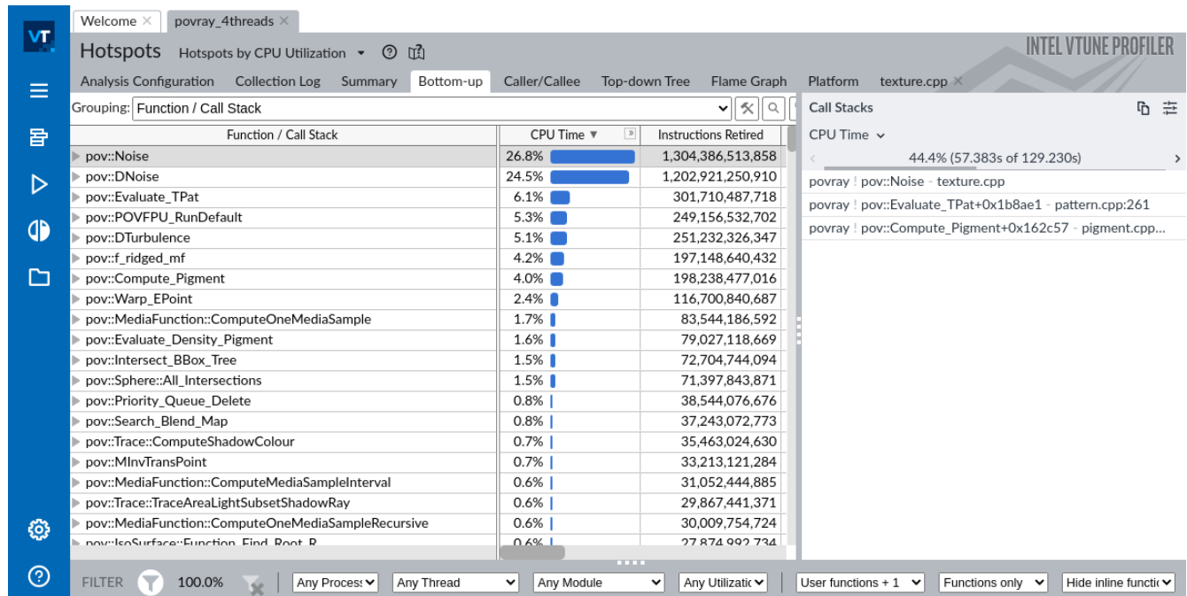
Figure 43: VTune 对 povray 内置基准测试的热点视图。
