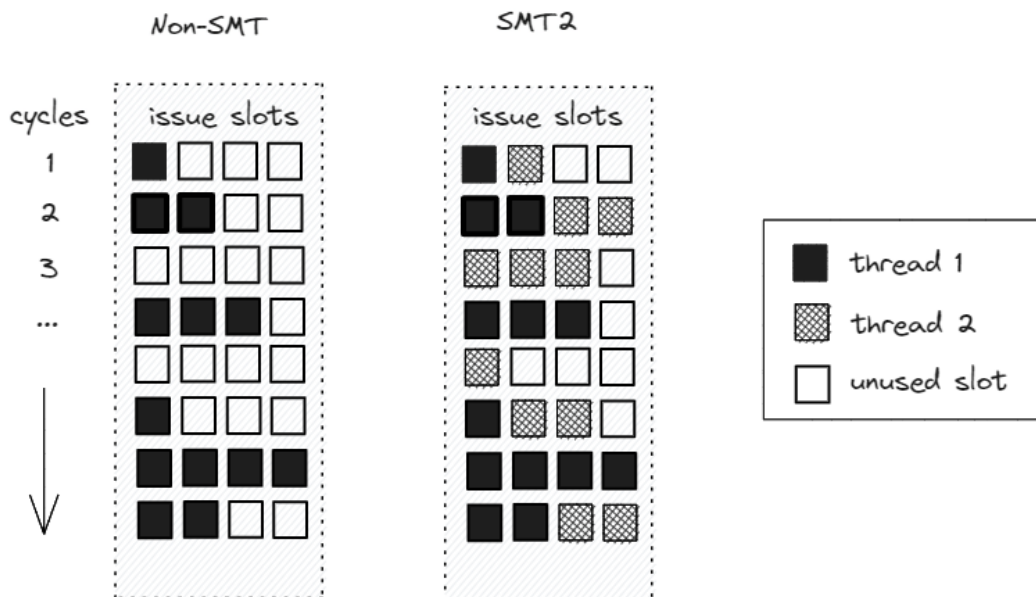
Figure 13: 在 4 宽度非 SMT 和 4 宽度 SMT2 处理器上的执行。
