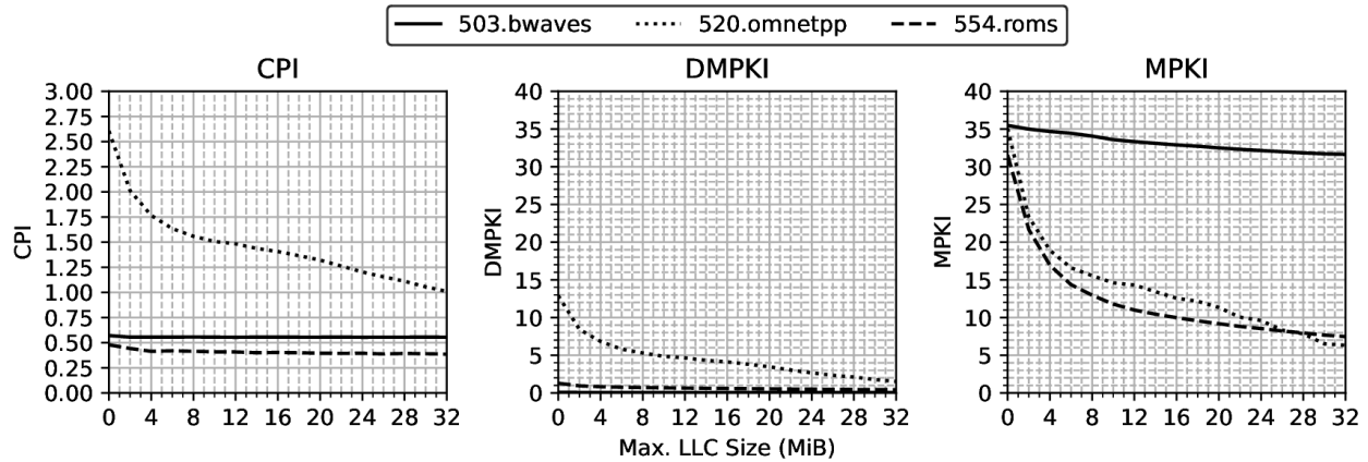
Figure 74: 随着 LLC 分配限制增加 (2 MiB 步长), CPI, DMPKI 和 MPKI.
