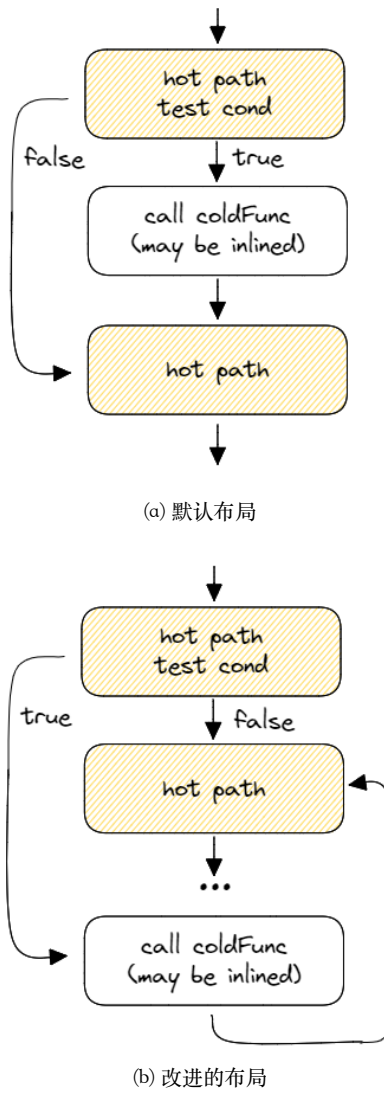
Figure 68: 上面代码片段的两种机器代码布局版本。
