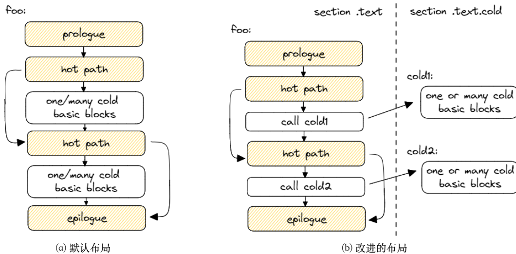
Figure 70: 将冷代码拆分到单独的函数中。
