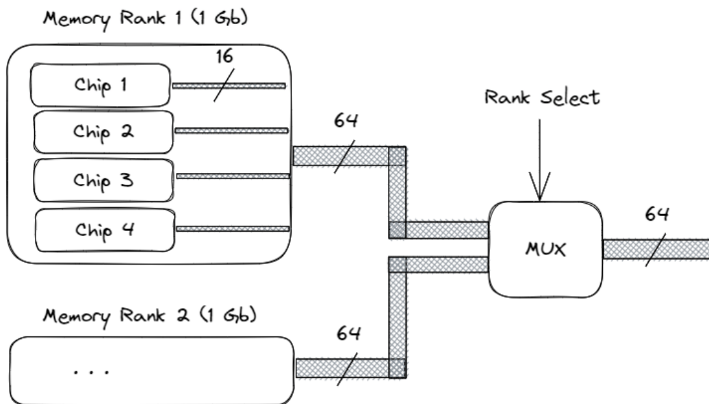
Figure 15: 2Rx16 双 rank DRAM DDR4 模块，总容量 2GB 的组织。
