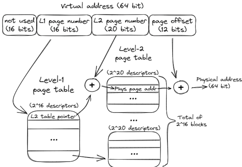
Figure 19: 2 级页表示例
