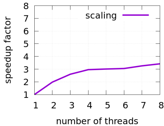
(a) 使用不同线程数量的性能扩展。
