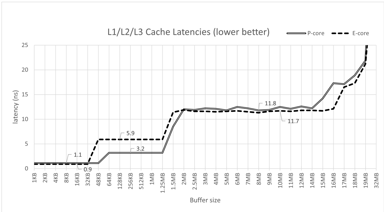
Figure 26: 在 Intel Core i7-1260P 上使用 mlc 工具测量的 L1/L2/L3 缓存读取延迟，启用了大页。
