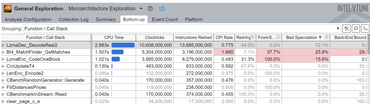
Figure 47: “微架构探索”自下而上视图。
