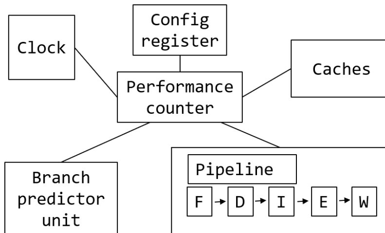
Figure 24: 带有性能监控计数器的 CPU 的简化视图。
