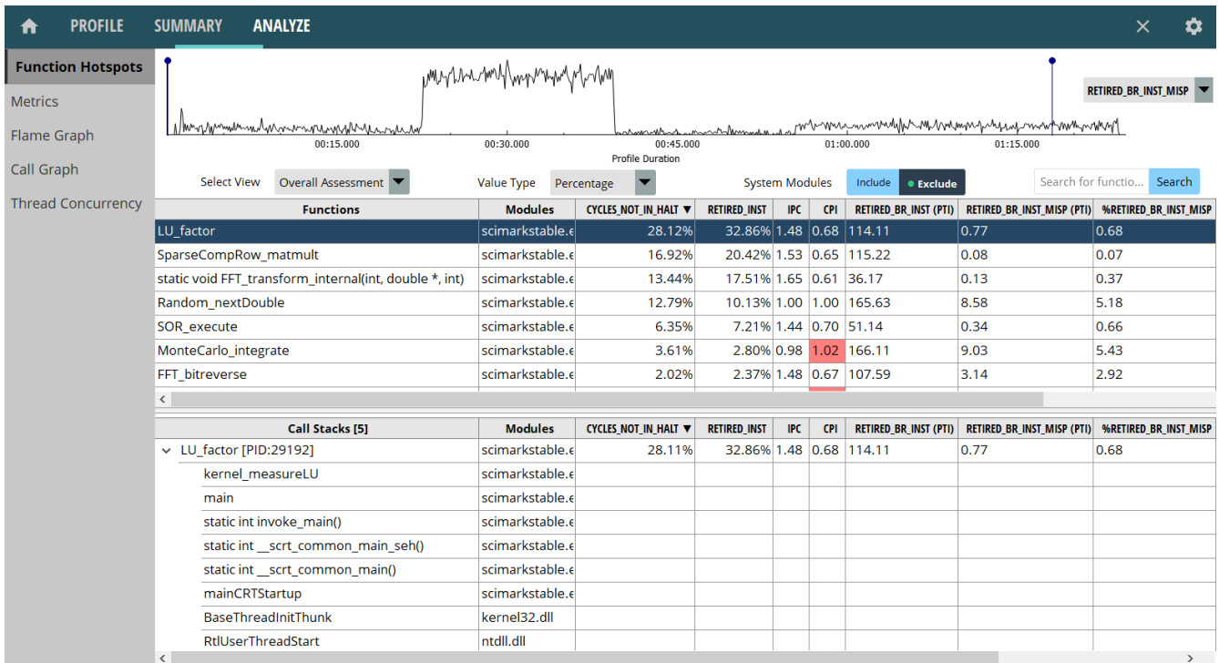
Figure 49: uProf 的函数热点视图。
