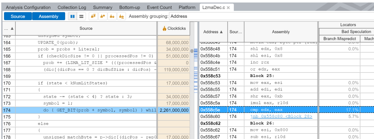
Figure 48: “微架构探索”源代码和汇编视图。
