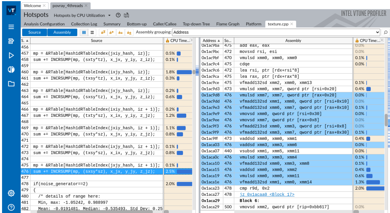
Figure 44: VTune 对 povray 内置基准测试的源代码视图。
