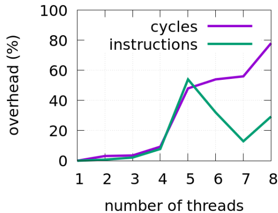
(b) 使用不同线程数量的开销。
