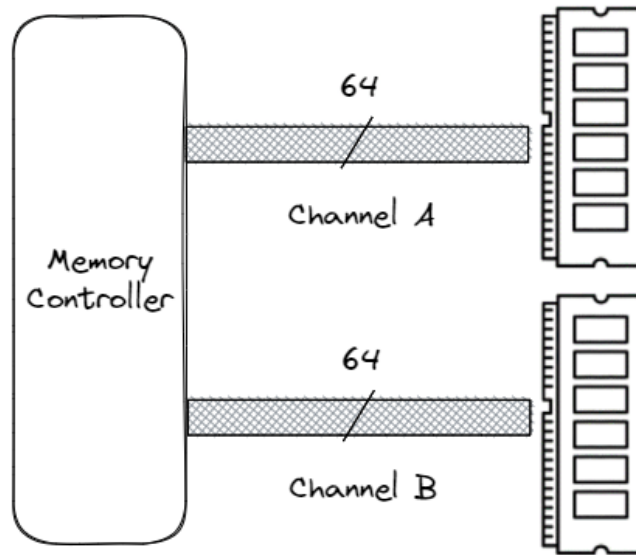
Figure 16: 双通道 DRAM 设置的组织。
