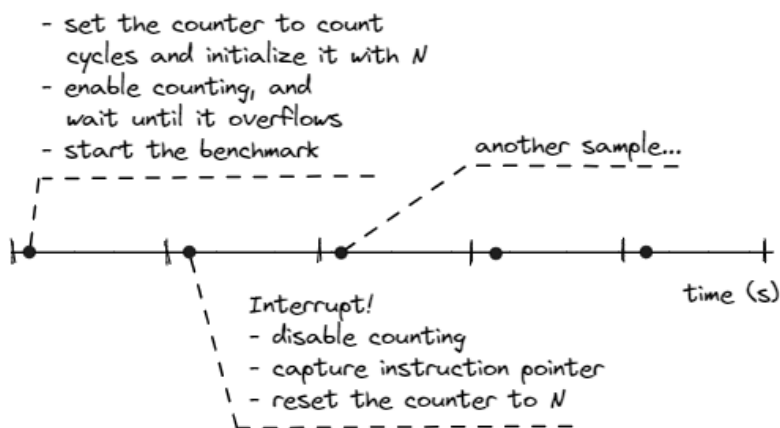
Figure 31: 使用性能计数器进行采样
