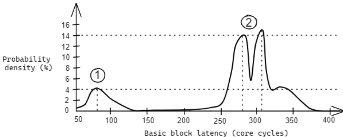
Figure 41: 基本块延迟的概率密度图，基本块起始地址为 0x400618
