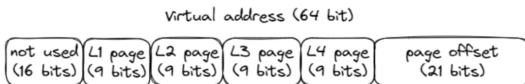
Figure 20: 指向 2MB 页面中数据的虚拟地址
