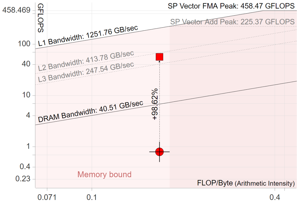
Figure 35: 在 Intel NUC 工具包 NUC8i5BEH 上使用 clang 10 编译器对矩阵乘法进行了 Roofline 分析
