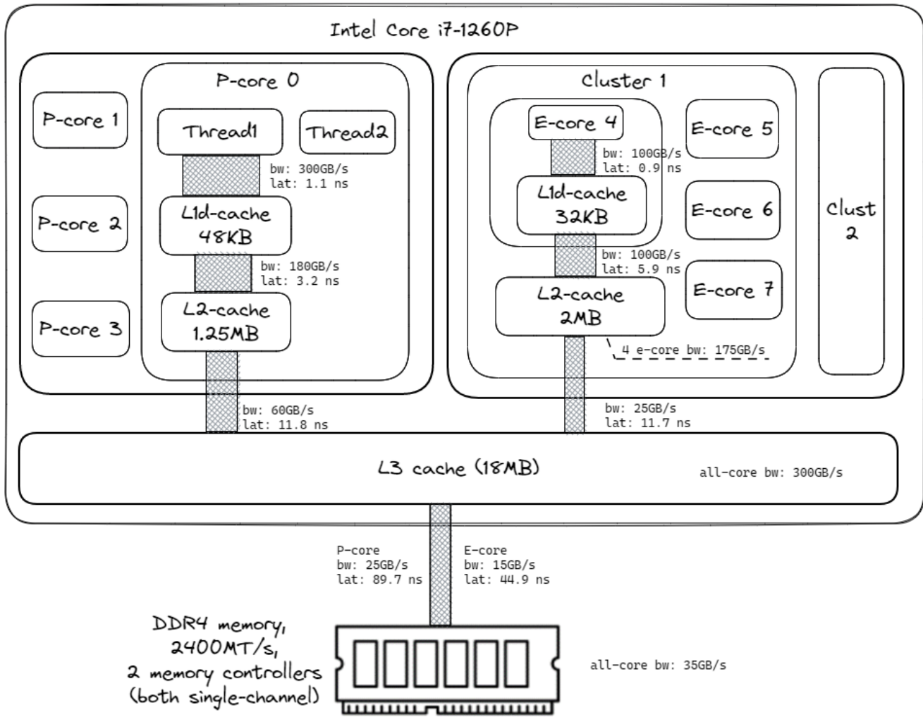
Figure 27: Intel Core i7-1260P 内存层次结构的块图和外部 DDR4 内存。
