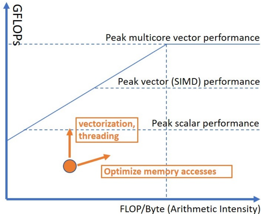
Figure 34: Roofline 性能模型
