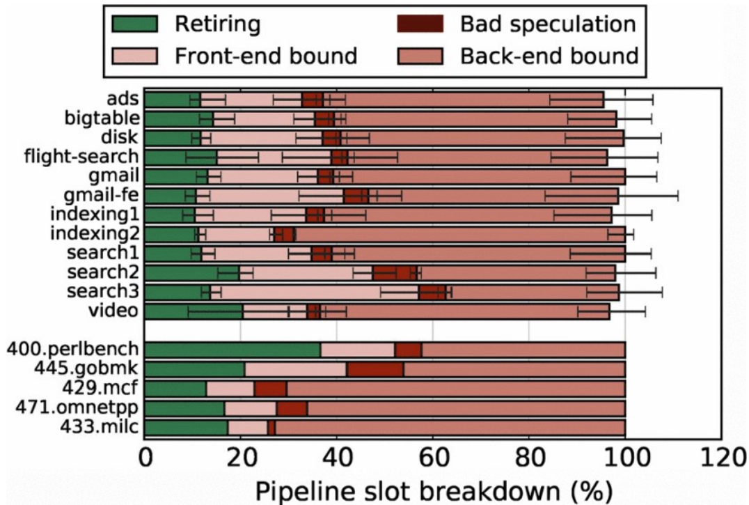
Figure 40: 谷歌数据中心工作负载的 TMA 分解以及几个 SPEC CPU2006 基准, © Image from [Kanev et al., 2015]
