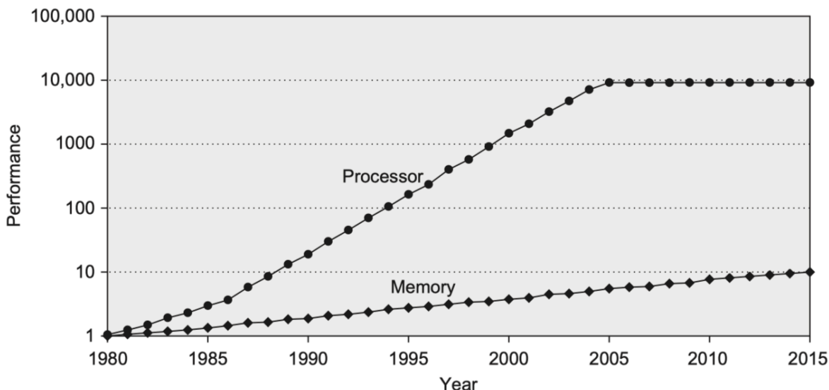
Figure 62: 内存和处理器之间性能差距。© 图片来自 [Hennessy & Patterson, 2017]。
