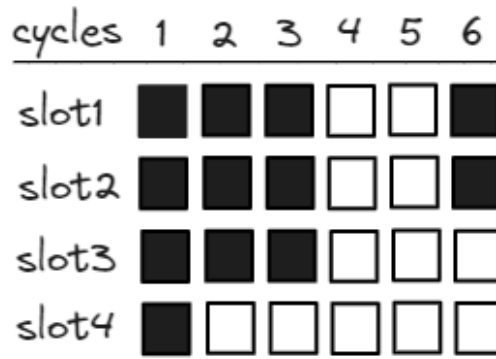
Figure 25: 4 宽 CPU 的流水线图
