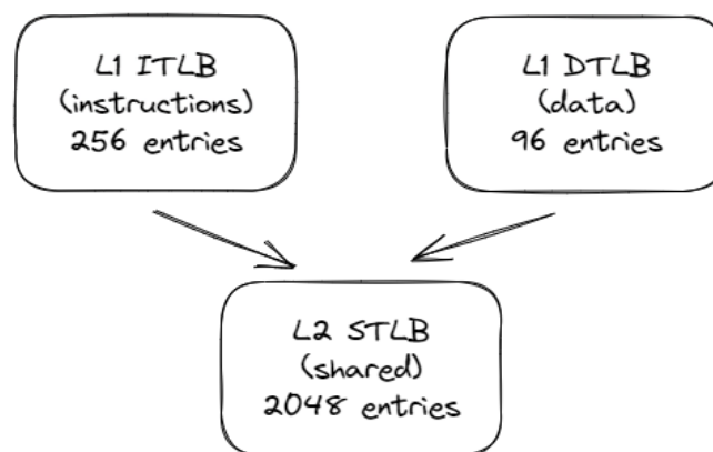
Figure 22: Golden Cove 的 TLB 层次.
