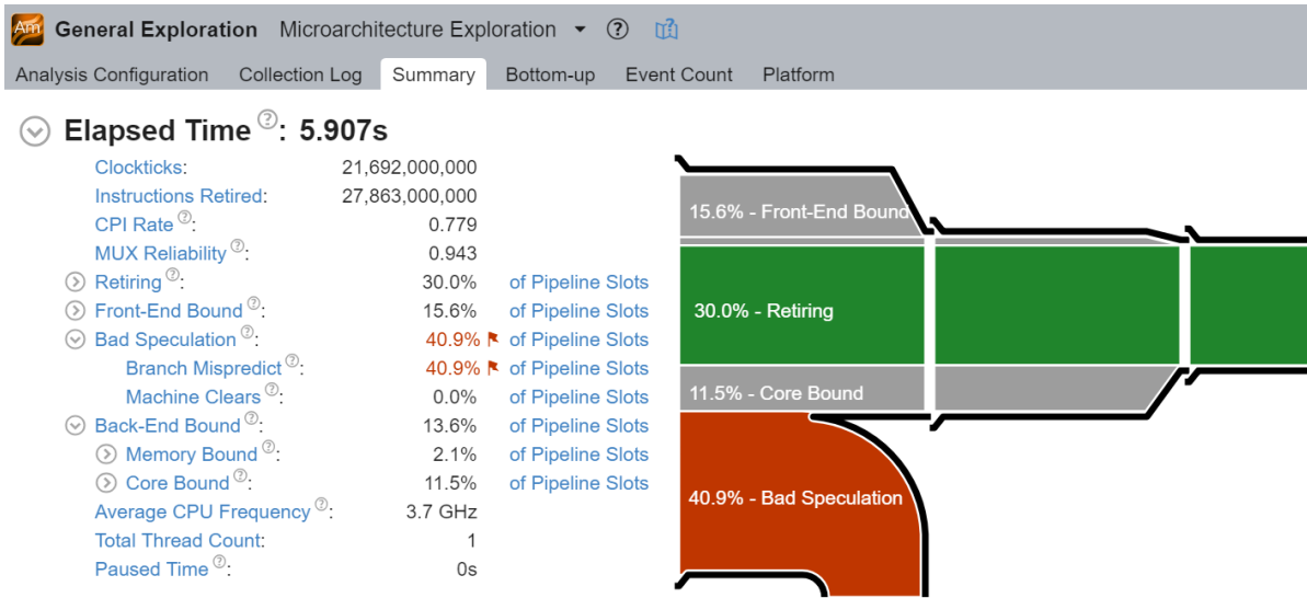
Figure 46: Intel VTune Profiler 中的“微架构探索”分析。
