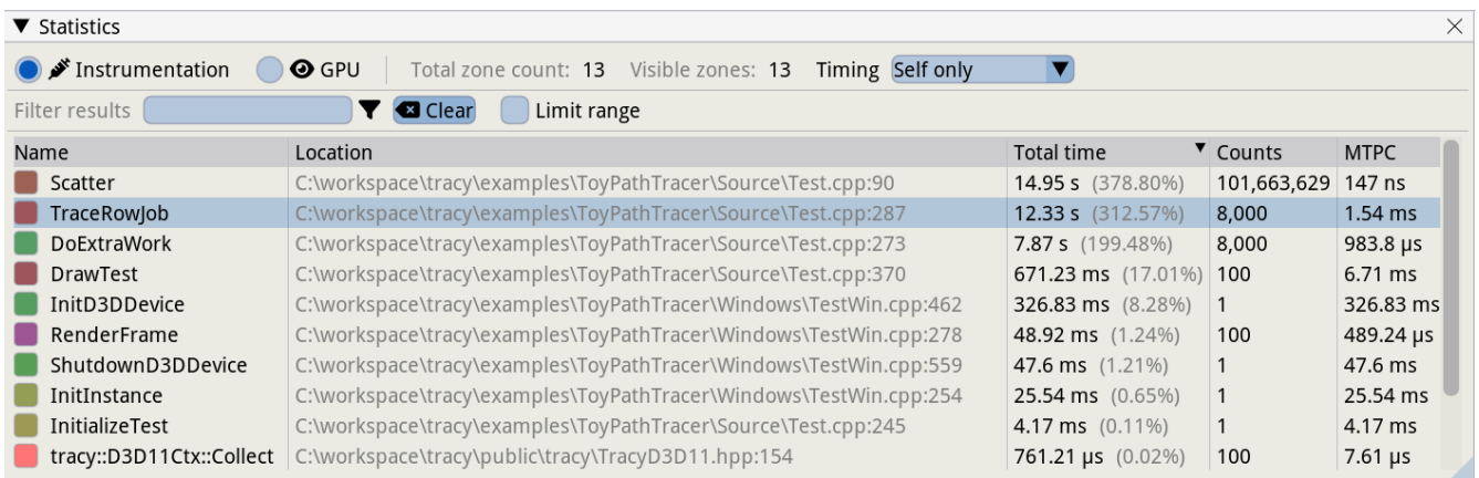
Figure 59: Tracy 函数统计数据.
